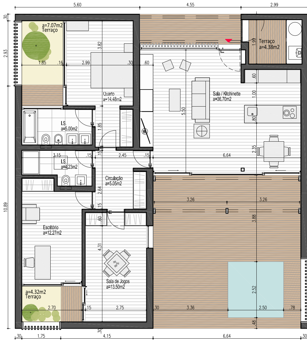
planta piso 0 . esc 1.100
